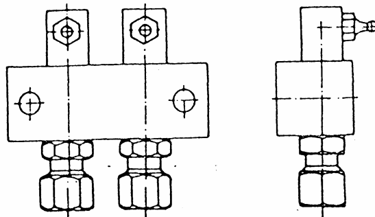
Nippelblok 2 smeernippels
