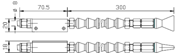
SPROEIER met plat mondstuk (trage voeding)
