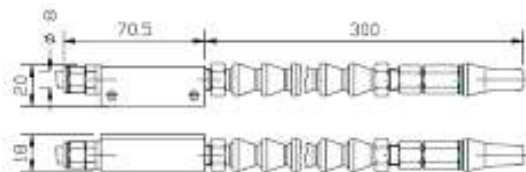
SPROEIER met conisch mondstuk (snelle voeding)
