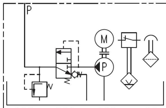
Hydraulisch plan
