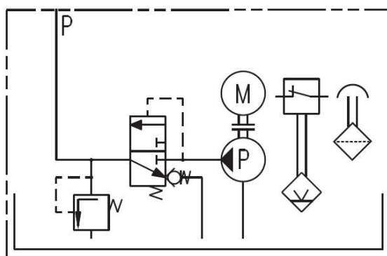
Hydraulisch plan
