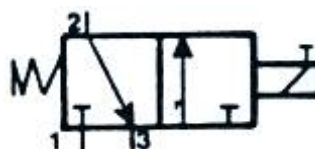
Type 3.04.18 Normaal gesloten
