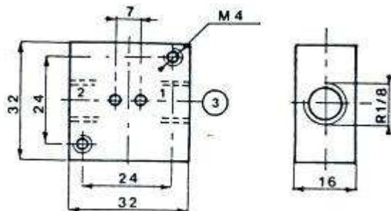
Rechte doorgang (type 3.00.04.00) (extra uitvoering)
