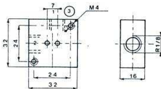
Doorgang haaks 90° (type 3.00.04.90) (standaarduitvoering)
