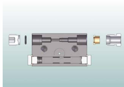
SEZIONE B-B
