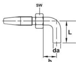
3 – INSERTO A 90°
