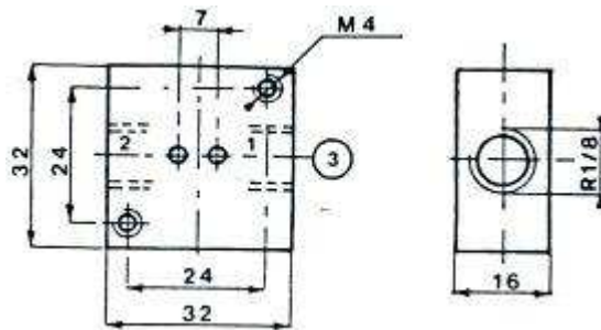
Straight flow path (type 3.00.04.00)
