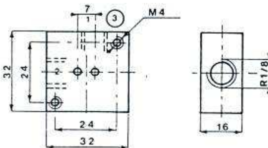
Perpendicular flow path (type 3.00.04.90)
