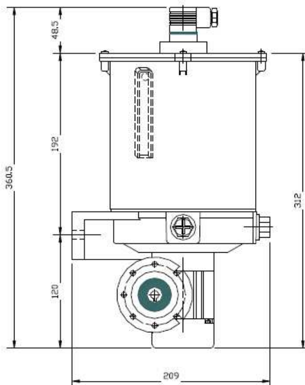
ABMESSUNGEN
